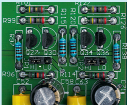
Переместив перемычки, можно изменить коэффициент усиления с 66 дБ на 60 дБ
